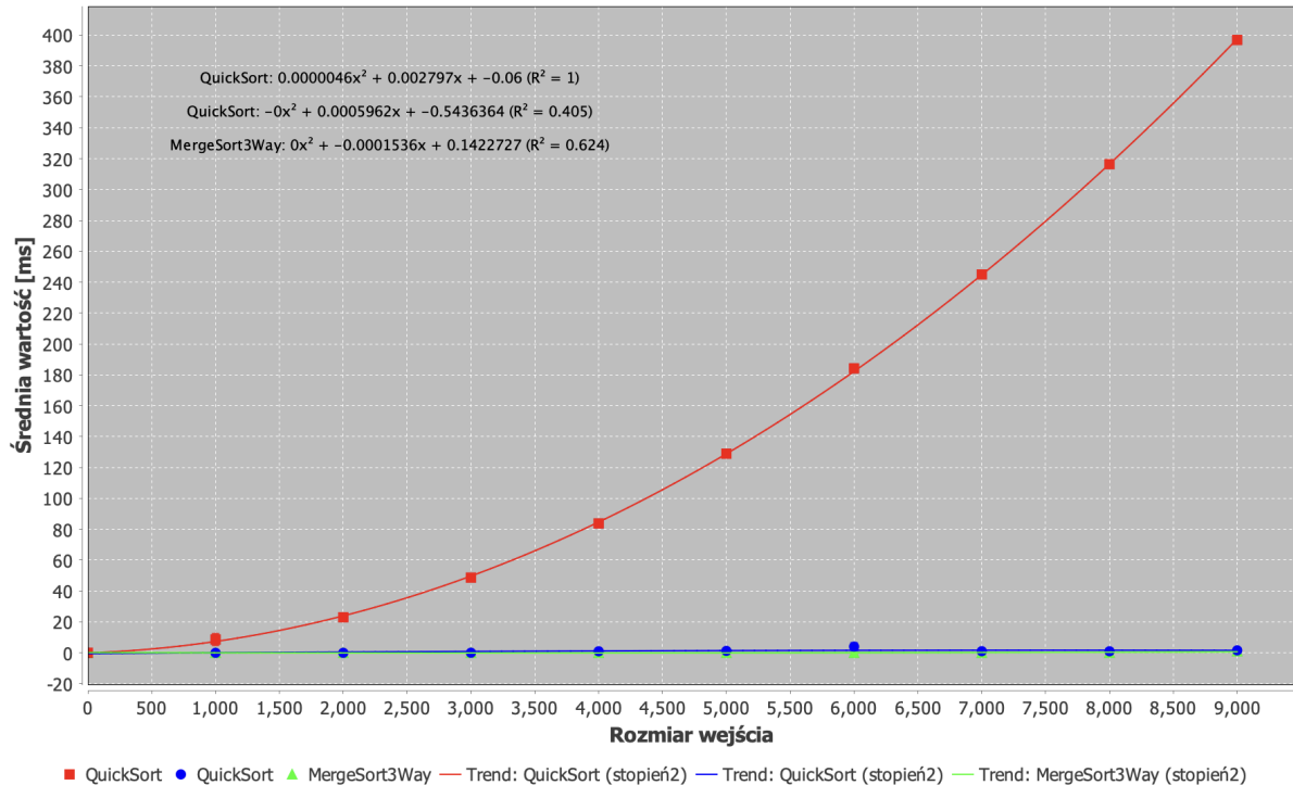
Wykres AiSD
