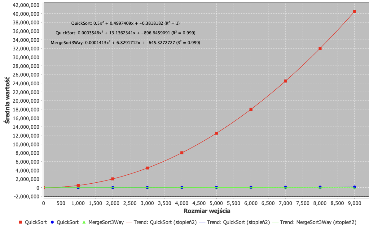
Wykres AiSD
